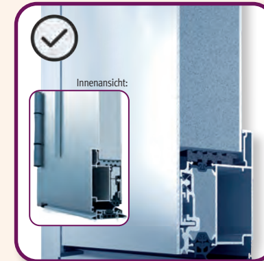
Außenansicht Aufsatzfüllung einseitig [Ud-Wert \leq 1,2 \text{ /m}^2\text{K} ]
